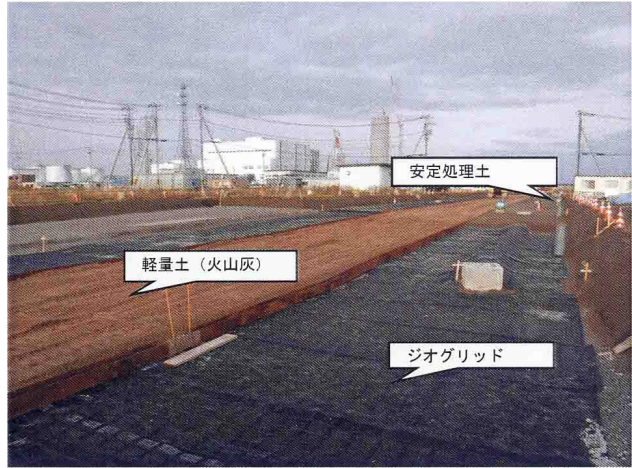
詳細(ジオグリッド、軽量土、安定処理度)
