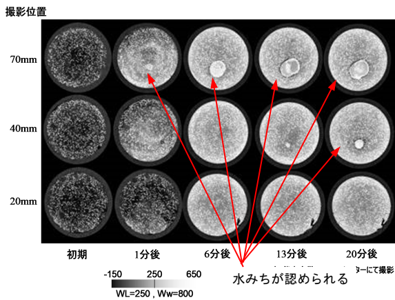
目詰まり試験結果(ジオテキ無)
