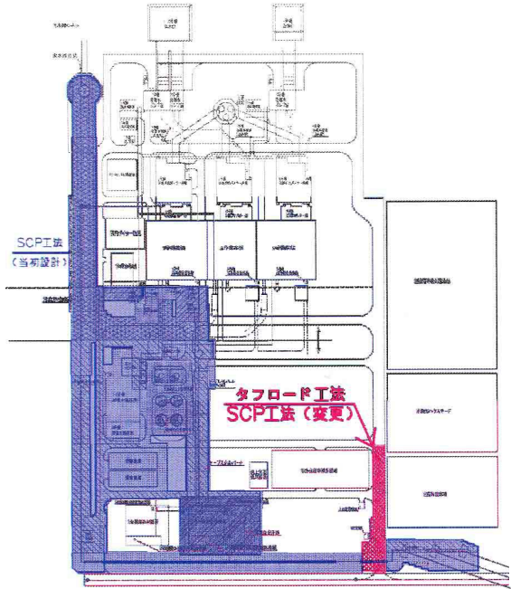
地盤改良計画
