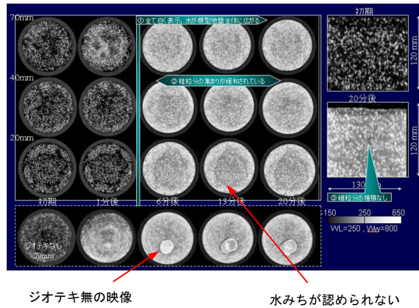
目詰まり試験結果(ジオテキ有)
