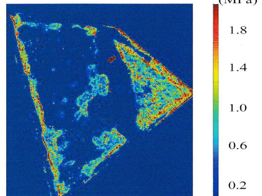
キャッピングの応力分布
