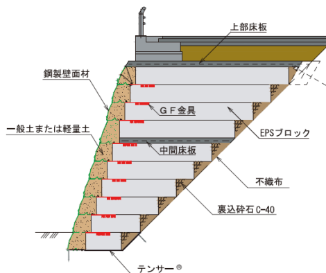
標準断面構造
