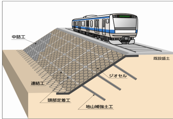
新用途 (RRS®工法) の概要
