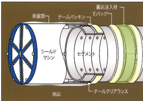
Eバッグ工法の概念
