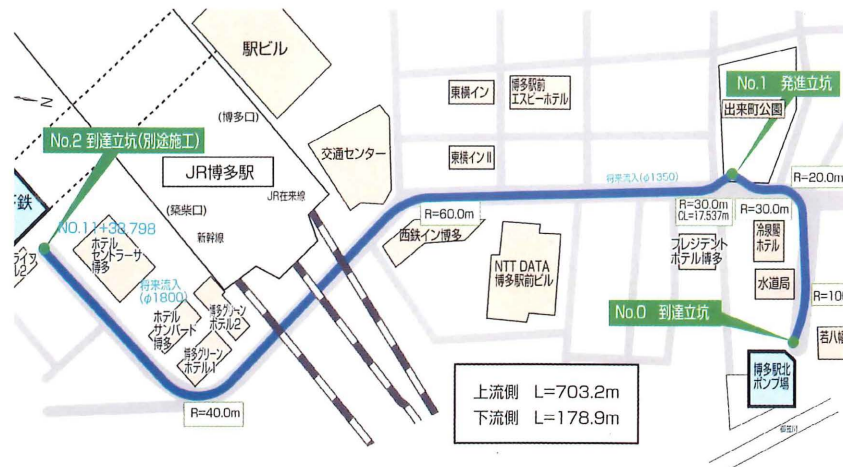
工事路線平面
