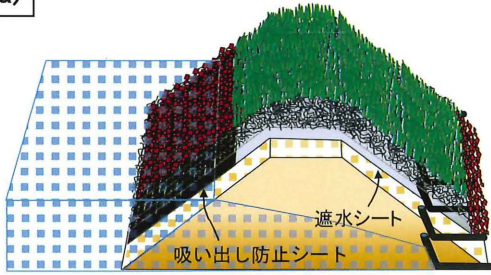
斜面安定のための表層被覆
