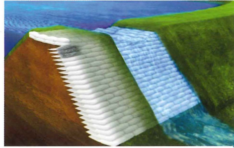
土嚢を用いたため池補強
