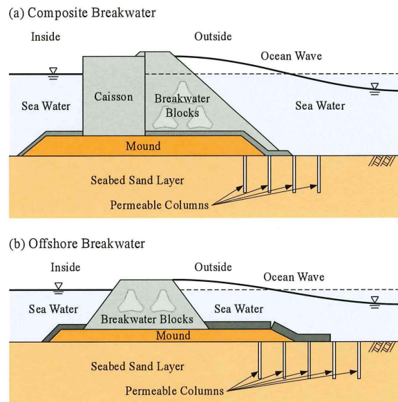
透水性コラム工法の適用例 (a) 混成防波堤、(b) 離岸堤
