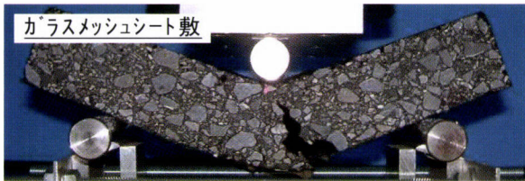
各強化シート敷設供試体のクラック発生状況
