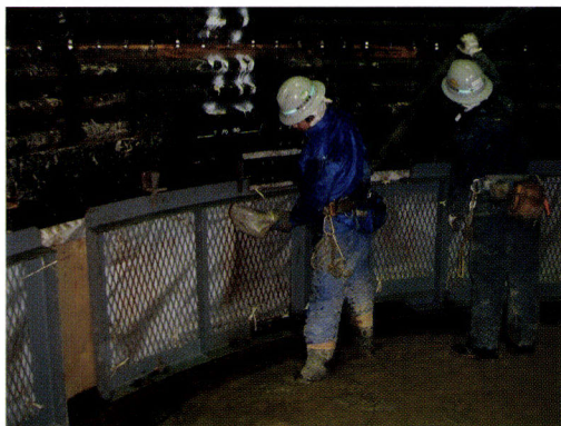
袋体へのモルタル充填状況
