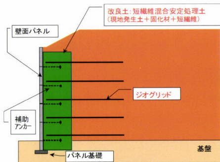
工法概念図
