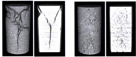
外観 内部 (a) 固化処理土
