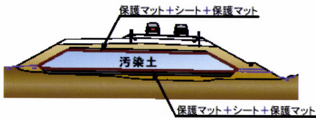
道路盛土遮水工封じ込めの概要
