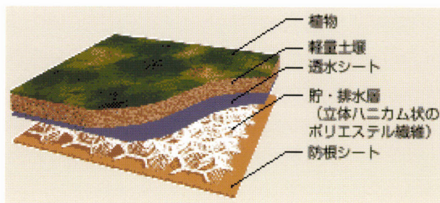
屋上緑化工法(薄層緑化)の概要
