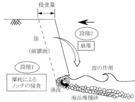
海岸侵食のメカニズムに関する模式図
