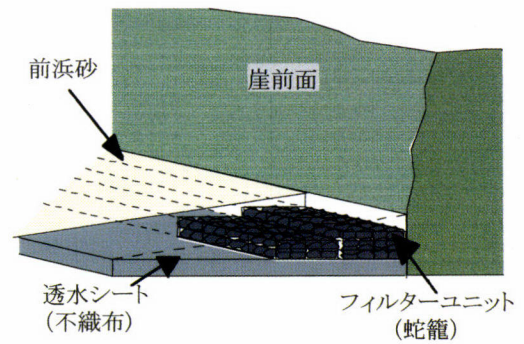
ジオシンセティックスを用いた 有効な侵食防止工法の一例
