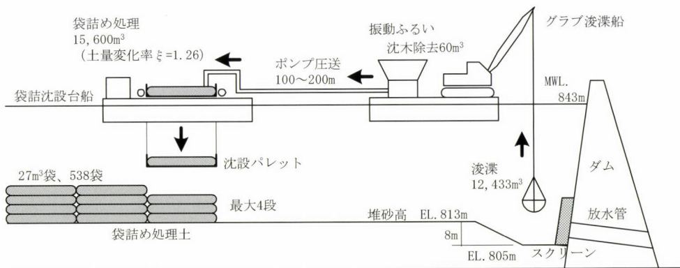
施工フロー
