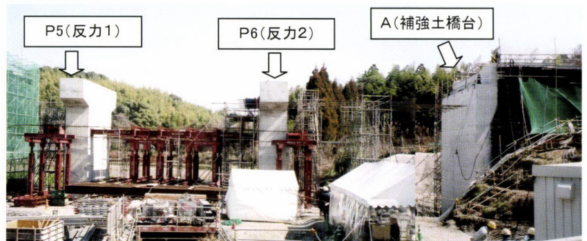
載荷試験装置の設置状況
