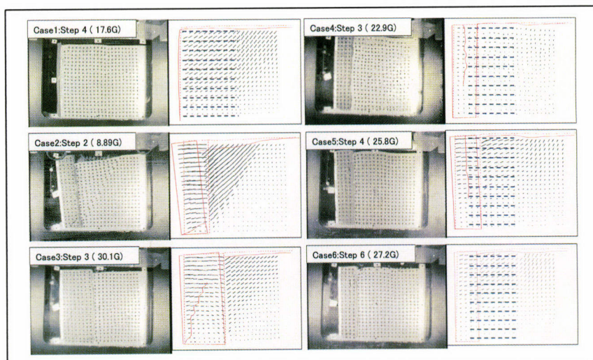
各ケースの振動台実験最終状況と変位ベクトル図
