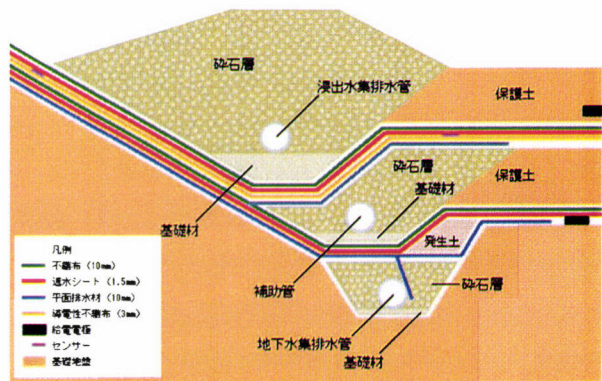
集排水管設置構造
