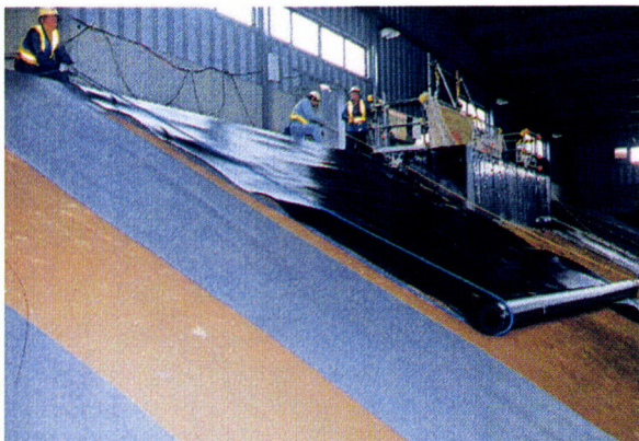
遮水シート施工状況
